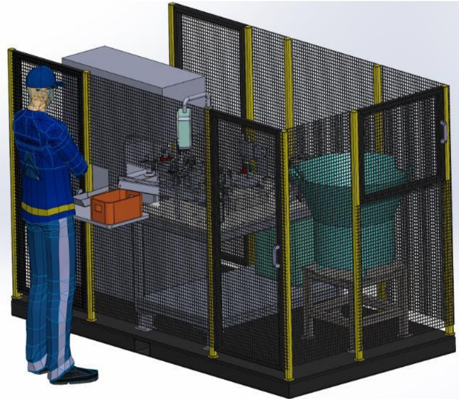
DÖNER TABLALI BESLEME VE PRES OTOMASYON SİSTEMİ
