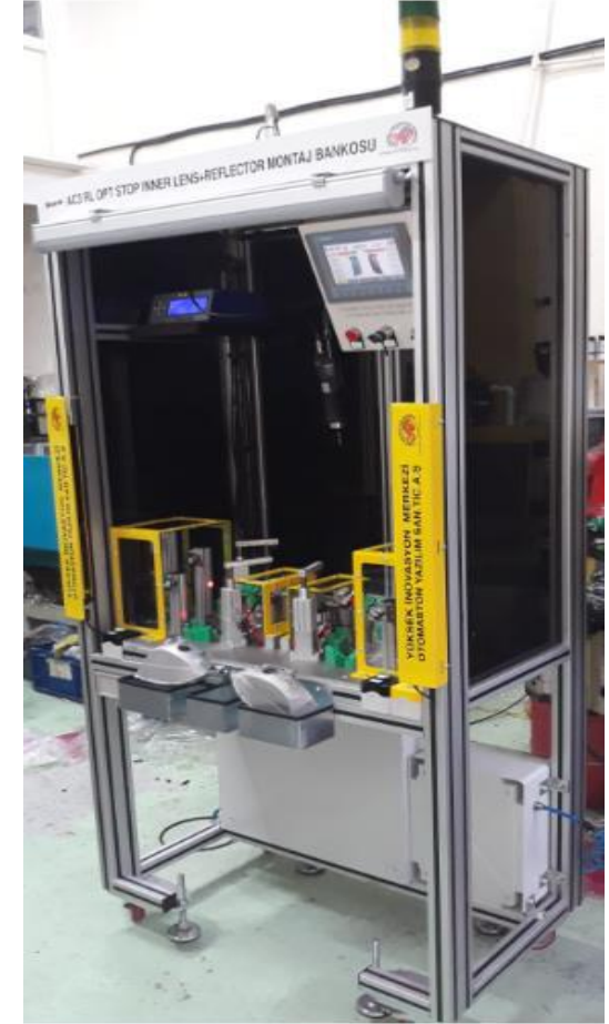
AC3 PROJECT POKA-YOKELİ , ELEKTRİKLİ TORKLU SIKICILI MONTAJ BANKOSU
