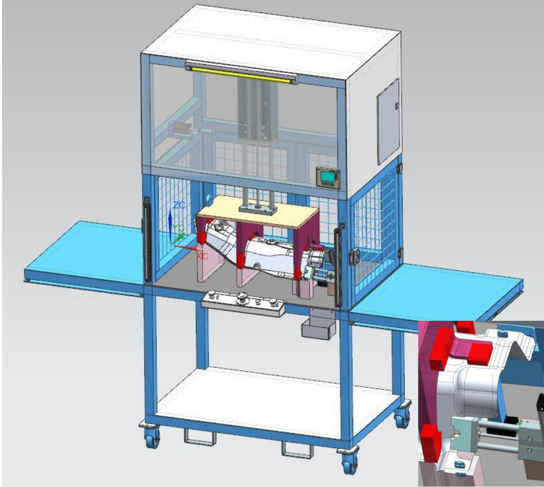
HYUNDAI PROJESİ OTOMATİK KLİPS ÇAKMA MAKİNASI
