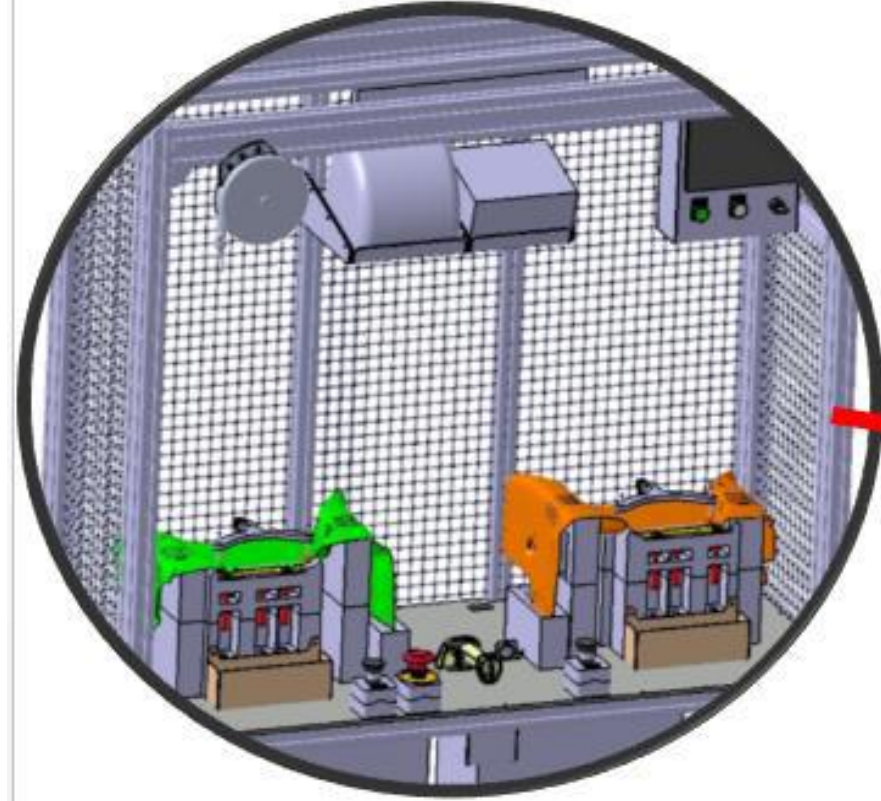
ELEKTRİKLİ SIKICILI VE BARKOD OKUYUCULU POKA-YOKE MASASI
