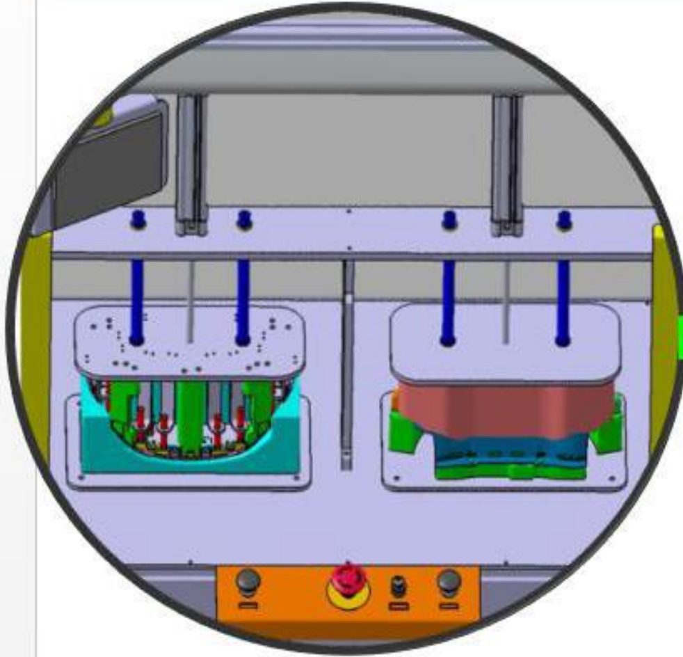
GÖSTERGE ÇERÇEVESİ PLASTİKLERİ MONTAJ BANKOSU
