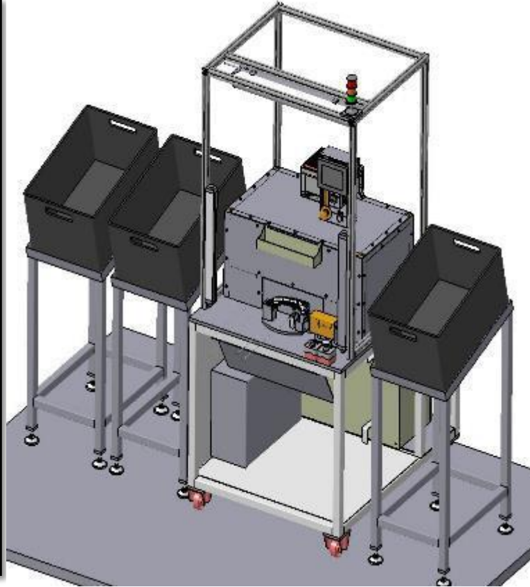
RENAULT BJA PROJECT KAPI KOLU POKA-YOKELİ MONTAJ BANKOSU Varlık , Pozisyon ve Montaj Kontrol Poka-Yokesi
