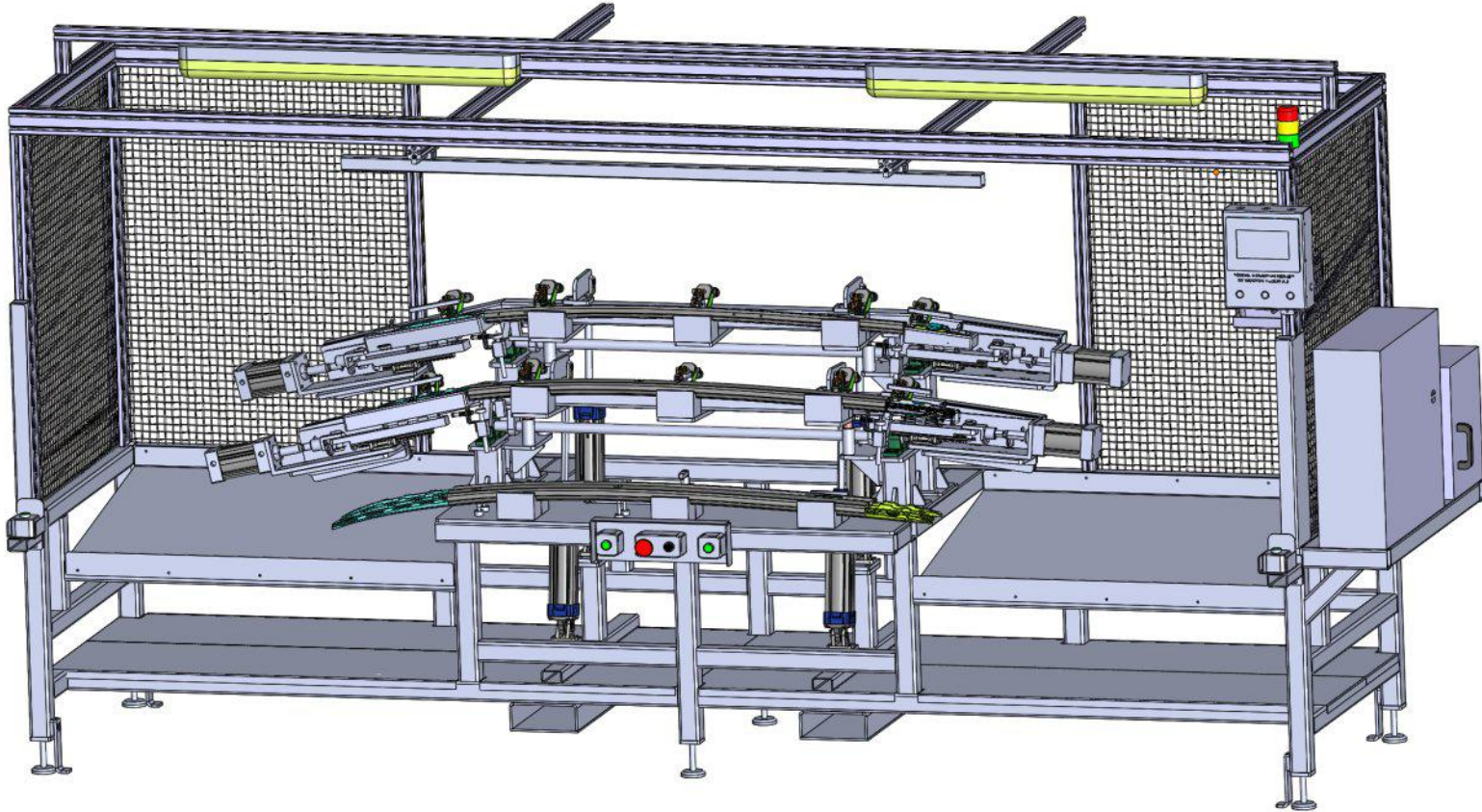
356 PROJECT PORTBAGAJ MONTAJ MAKİNASI
