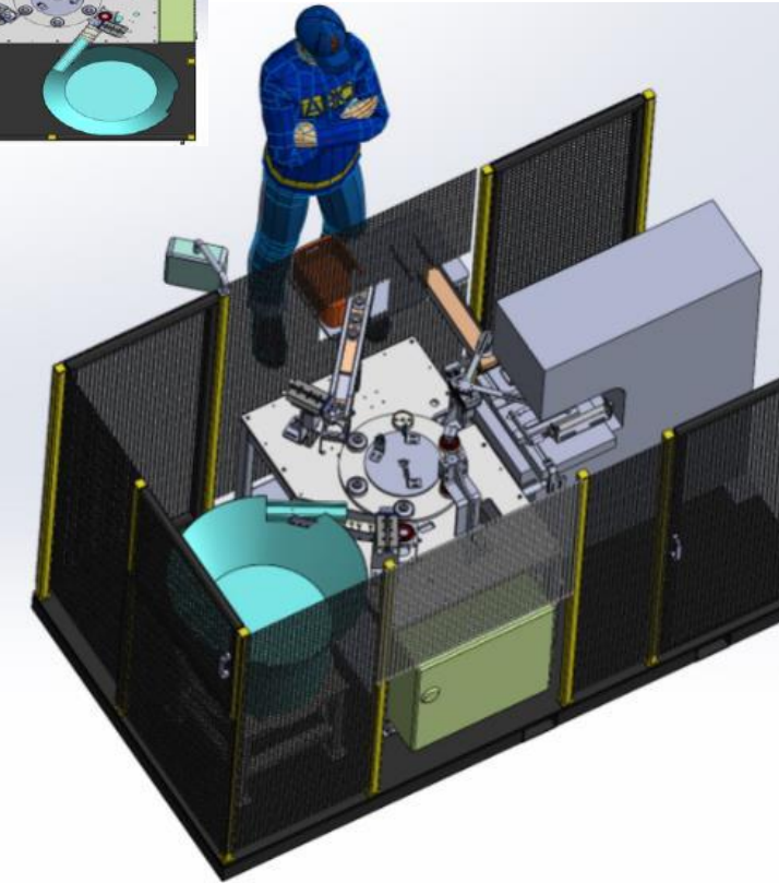
DÖNER TABLALI BESLEME VE PRES OTOMASYON SİSTEMİ
