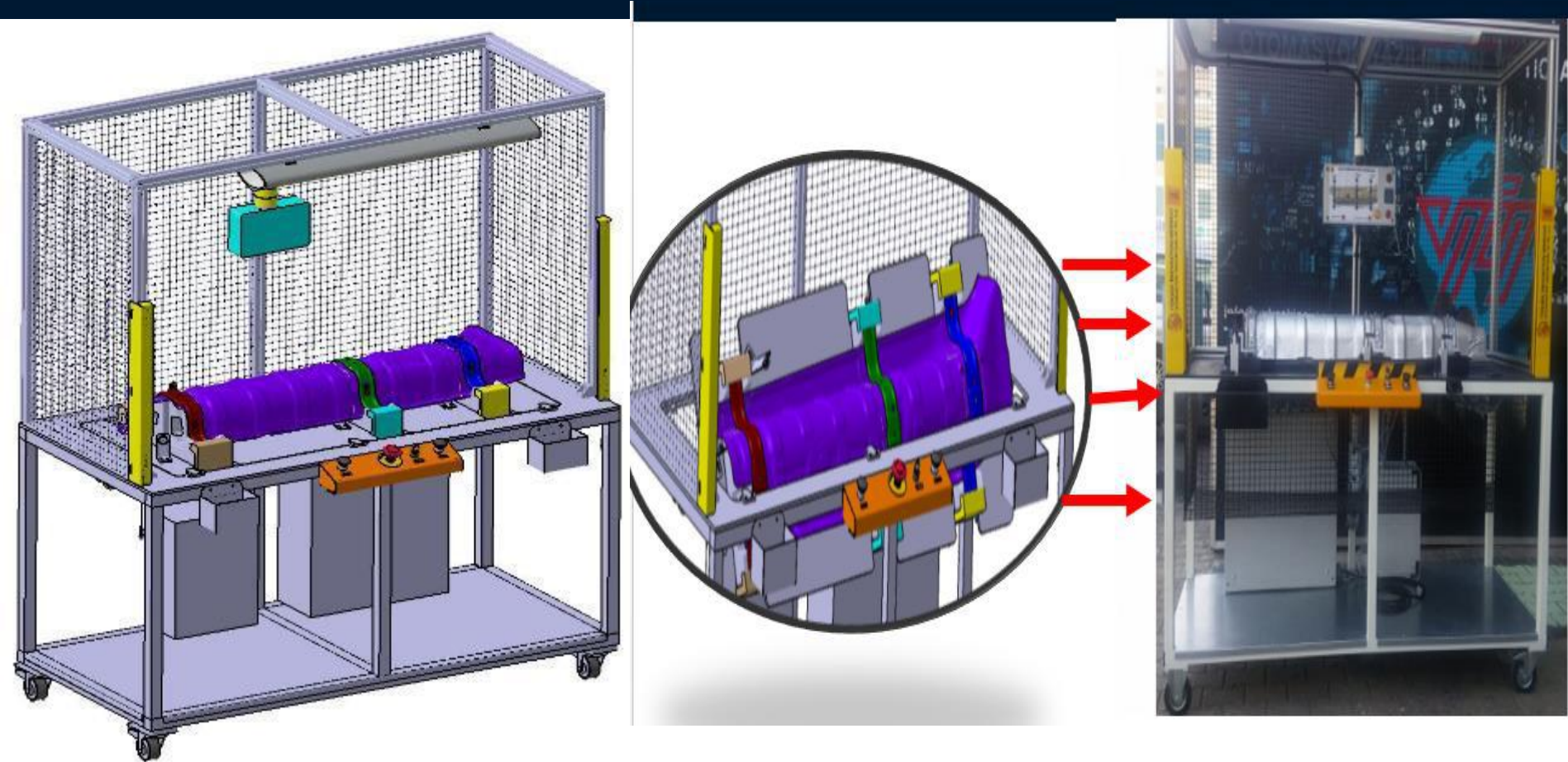
TOYOTA PROJECT PNÖMATİK DÖNER SİSTEMLİ PERÇİN ÇAKMA VE MONTAJ KONTROL BANKOSU Otomasyonlu Perçin çakma ve Parça Kontrolü
