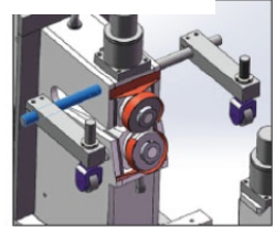
OPSİYONEL IDK-5 için Flanşlama Etek Bükme Destek Aparatı
