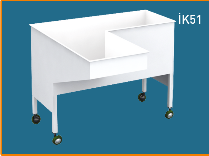
SAC KOLLU MAKİNASI TEKNEŞİ TEKERLEKLİ En / W: 45 cm BOY / L:95 cm YÜKS / H: 76 cm
