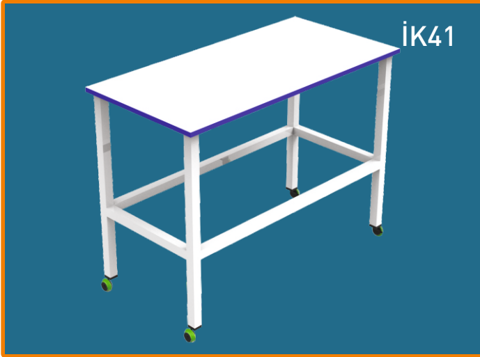
TEKERLEKLİ MAKİNA YAN SEHPASI En / W: 50 cm BOY / L: 110 cm YÜKS / H: 76 cm
