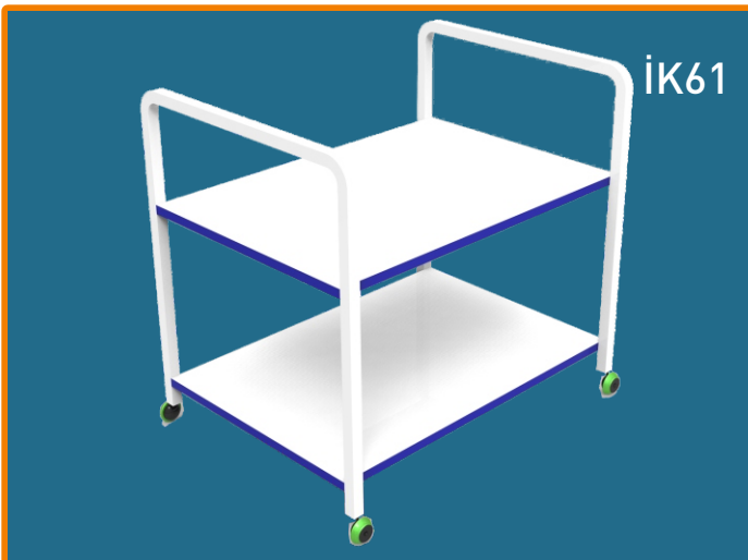
KOLİ TAŞIMA ARABASI En / W: 50 cm BOY / L: 90 cm YÜKS / H: 80 cm
