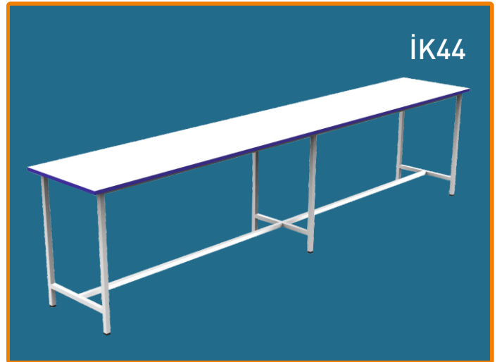
MAKİNA YANI BANT SEHPA En / W: 50 cm BOY / L: 250 cm YÜKS / H: 76 cm
