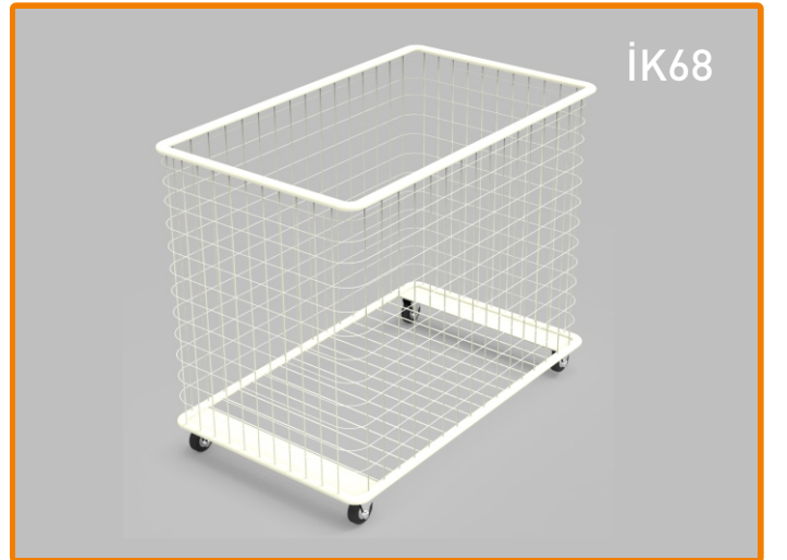
TEKERLEKLİ HASIR TEL SEPET En / W: 60 cm BOY / L: 90 cm YÜKS / H: 76 cm
