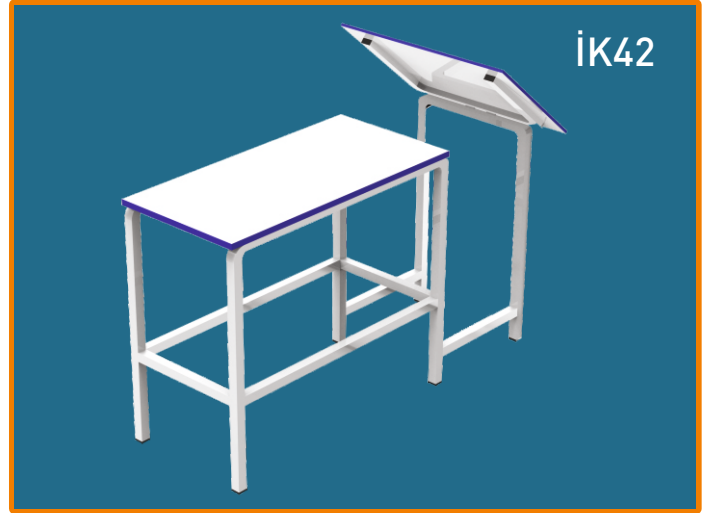
PASKARA YANI SEHPASI KAPAKLI En / W: 60 cm BOY / L: 132 cm YÜKS / H: 76 cm
