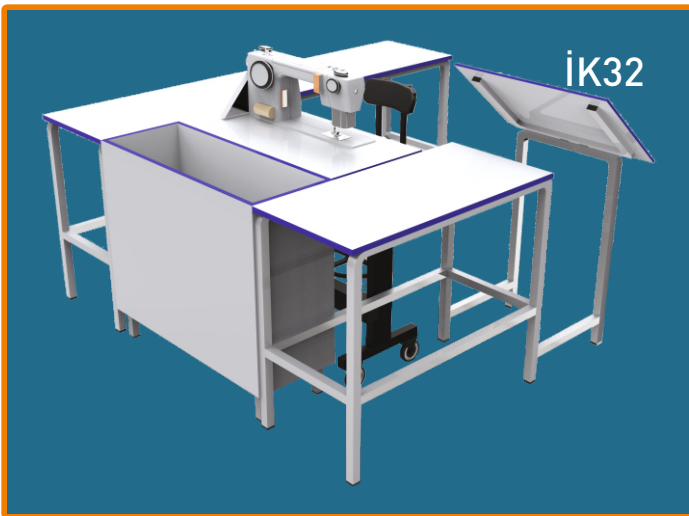
KAPAKLI SEHPA, SUNTALAM TEKNE VE SAĞ L SEHPA En / W: 180 cm BOY / L: 150 cm YÜKS / H: 76 cm
