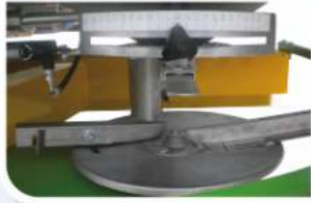
Hassas ve Çok Fonksiyonlu Serpme Ayarı Very precise fertilizing adjustment
