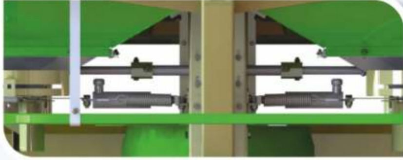
Hidrolik Açma ve Kapama Sistemi / Hydraulic Open and Close
