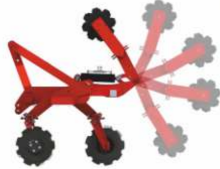
Opsiyonel Hidrolik Kontrollü Katlanır Merdane Optional Hydraulic Control / Folded Roller
