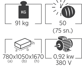
IUN 01 İPEK UN ELEME MAKİNESİ SIFT FLOUR MACHINE
