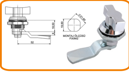
YAYLI PANO KİLİDİ (METAL KELEBEK)
