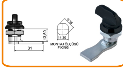
MİNİ YAYLI PANO KİLİDİ (STATİK BOYALI)
