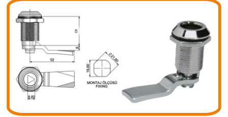
YAYLI PANO KİLİDİ (40 mm)
