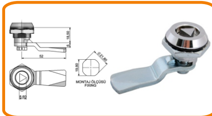
YAYLI PANO KİLİDİ (ÜÇGEN)
