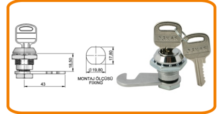
MANDALLI KİLİT (ŞİFRELE VE SEKMALİ)
