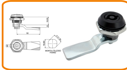
YAYLI PANO KİLİDİ STATİK BOYALI (DB)
