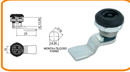
MİNİ YAYLI PANO KİLİDİ (TORNA VİDA BASLI STATİK BOYALI)
