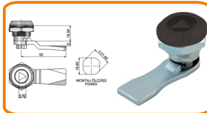
YAYLI PANO KİLİDİ STATİK BOYALI (ÜÇGEN)
