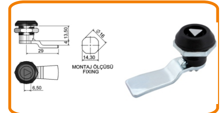
MİNİ YAYLI PANO KİLİDİ (PLASTİK ÜÇGEN)
