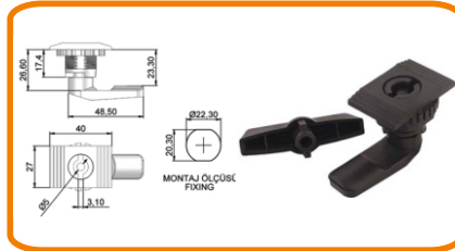
YAYLI PANO KİLİDİ (DÖRTGEN)
