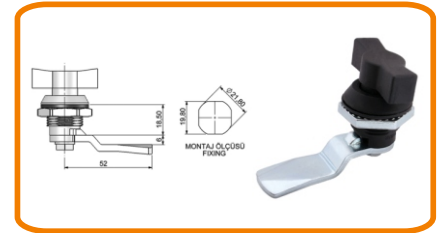
YAYLI PANO KİLİDİ (PLASTİK KELEBEK)
