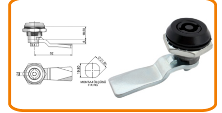
MİNİ YAYLI PANO KİLİDİ (PLASTİK DB)
