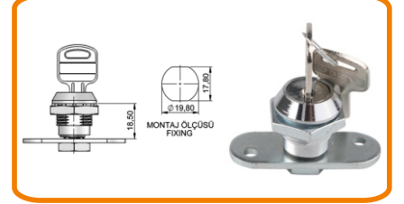
MANDALLI KİLİT (İSPANYOLET)
