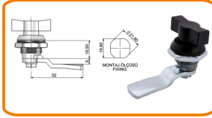
YAYLI PANO KİLİDİ STATİK BOYA (METAL KELEBEK)
