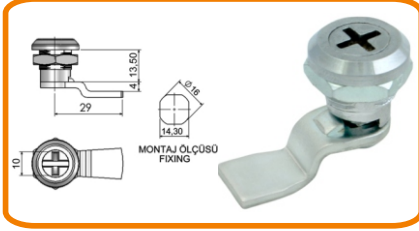
MİNİ YAYLI PANO KİLİDİ (TORNA VİDA BASLI)
