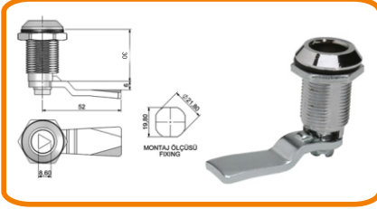
YAYLI PANO KİLİDİ (30 mm)
