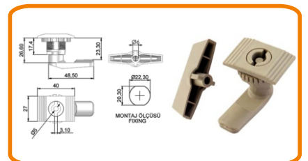
YAYLI PANO KİLİDİ (DÖRTGEN RAL-7032)
