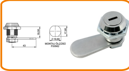
MANDALLI KİLİT (TORNA VİDA BAŞLI)
