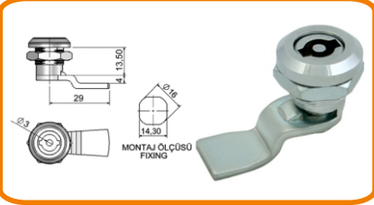
MİNİ YAYLI PANO KİLİDİ (DB)
