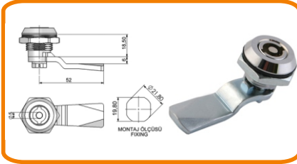
YAYLI PANO KİLİDİ (DB)
