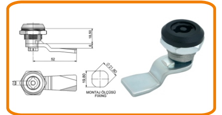
YAYLI PANO KİLİDİ (PLASTİK DB)
