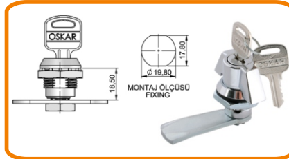
SİLİNDİR YAYLI PANO KİLİDİ (KELEBEK)
