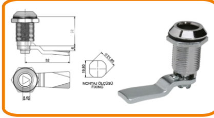
YAYLI PANO KİLİDİ (35 mm)
