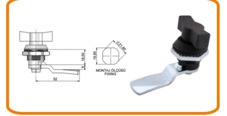
MİNİ YAYLI PANO KİLİDİ (PLASTİK KELEBEK)
