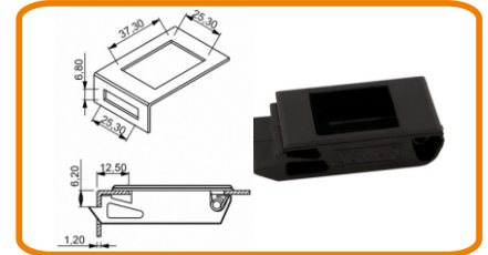
SÜRGÜ KİLİT (1.2mm)
