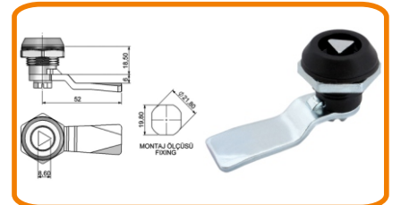
PLS. YAYLI PANO KİLİDİ (ZAMAK ÜÇGEN GÖBEKLİ)
