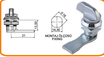
MİNİ YAYLI PANO KİLİDİ
