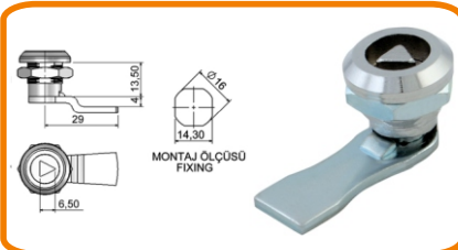
MİNİ YAYLI PANO KİLİDİ (ÜÇGEN)
