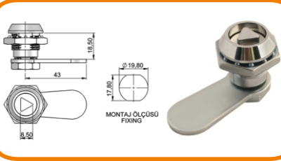
BİLYALI PANO KİLİDİ (ÜÇGEN)
