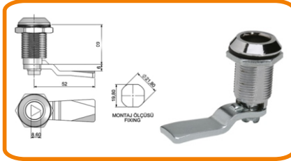
YAYLI PANO KİLİDİ (60 mm)
