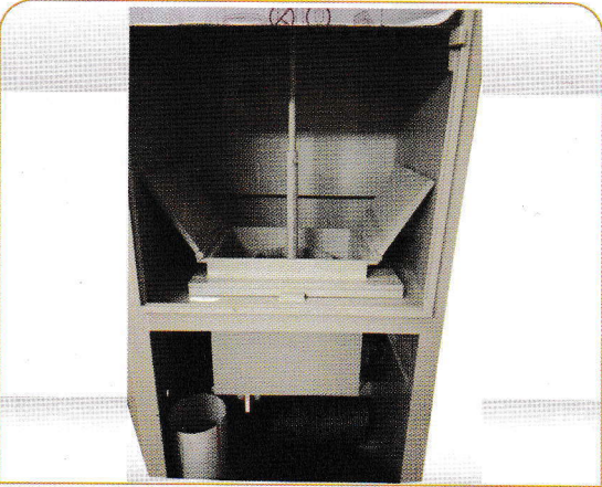
Demir ve Bakır Boşaltma Makinası (Hassas Mallar İçin)
