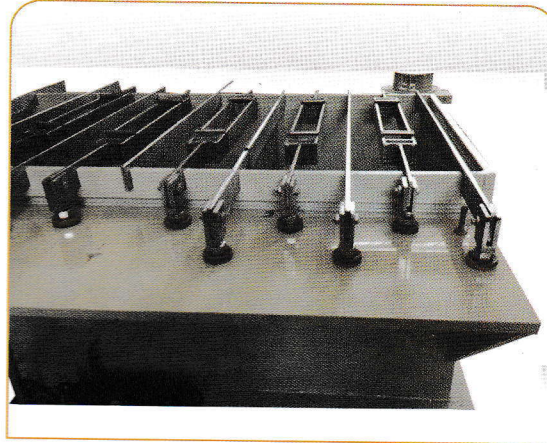
Gümüş Elektroliz
