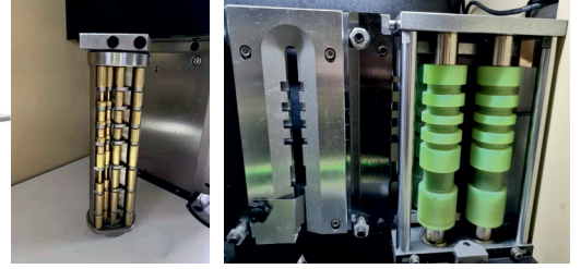
Alüminyum Malzeme için Özel Büküm ve Kesim Sistemi
