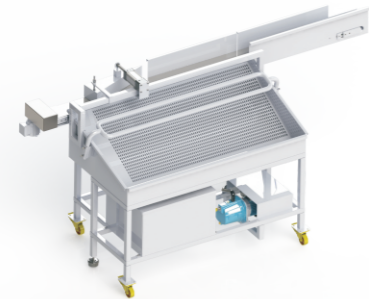
İstifleme ve Ayırma Ünitesi / Stowage-Separation Unit
