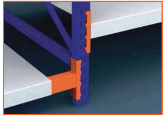
Ağır hizmet tip raf detayı
