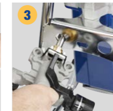
3 Pompayı gevşetmek ve kartuşu çıkarmak için şasi altıgen fitting kullanın
