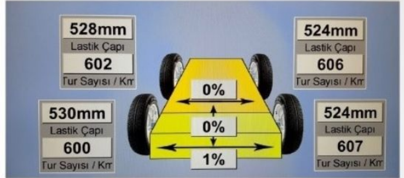
Tekerlek Çap ve Kilometredeki Tur Sayısı Ölçümü
