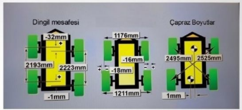
Aracın Çapraz Boyutları (Çapraz Şase Ölçümü)
