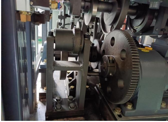
Dişli Şanzıman Yapısı
