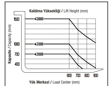
YÜK TABLOSU / LOAD CHART WS 1530
