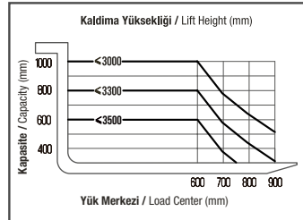
YÜK TABLOSU / LOAD CHART WS 1525
