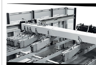
Üst seviyede hassasiyeti garanti eden tutucu sistemler
