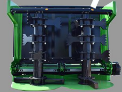
ÇİFT TEPSELİ VE TOKATLAMALI DAĞITICI SİSTEM
