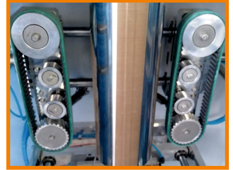
Film Çekme Sistemi
