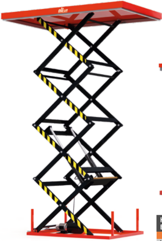
HW2000F Elektrikli Sabit Yük Platformu
