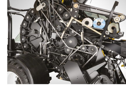
Merdaneli tip balya odası tasarımı
