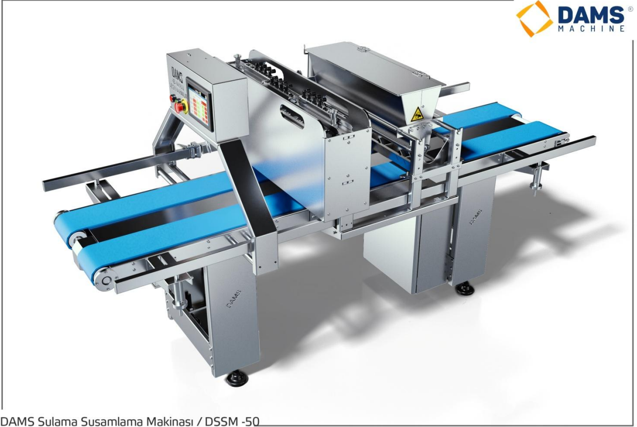
DAMS Sulama Susamlama Makinası / DSSM -50
