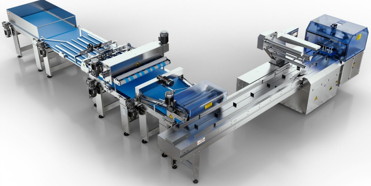
DAMS Gezer Çene Grup Paketleme Besleme Yarma / DGYR-50
