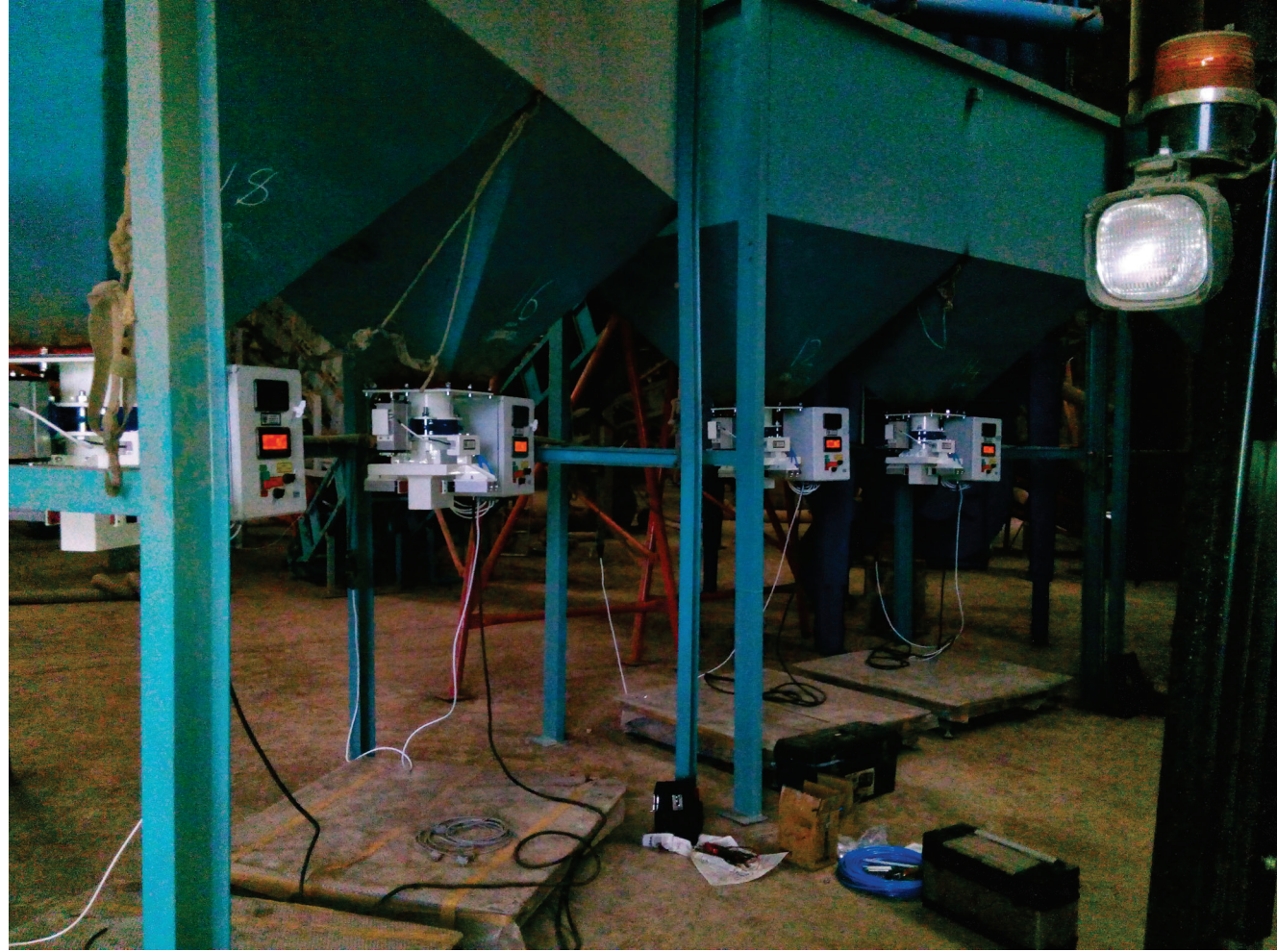
Maden Tozu için Serbest Akış Dolum Makinesi Uygulaması
